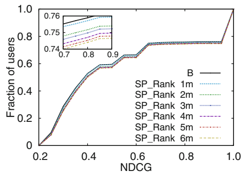
(d) NDCG distribution (SP_Rank).
